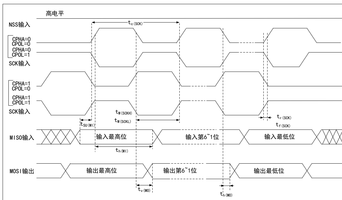
图17 SPI 时序图 — 主模式 (1)
