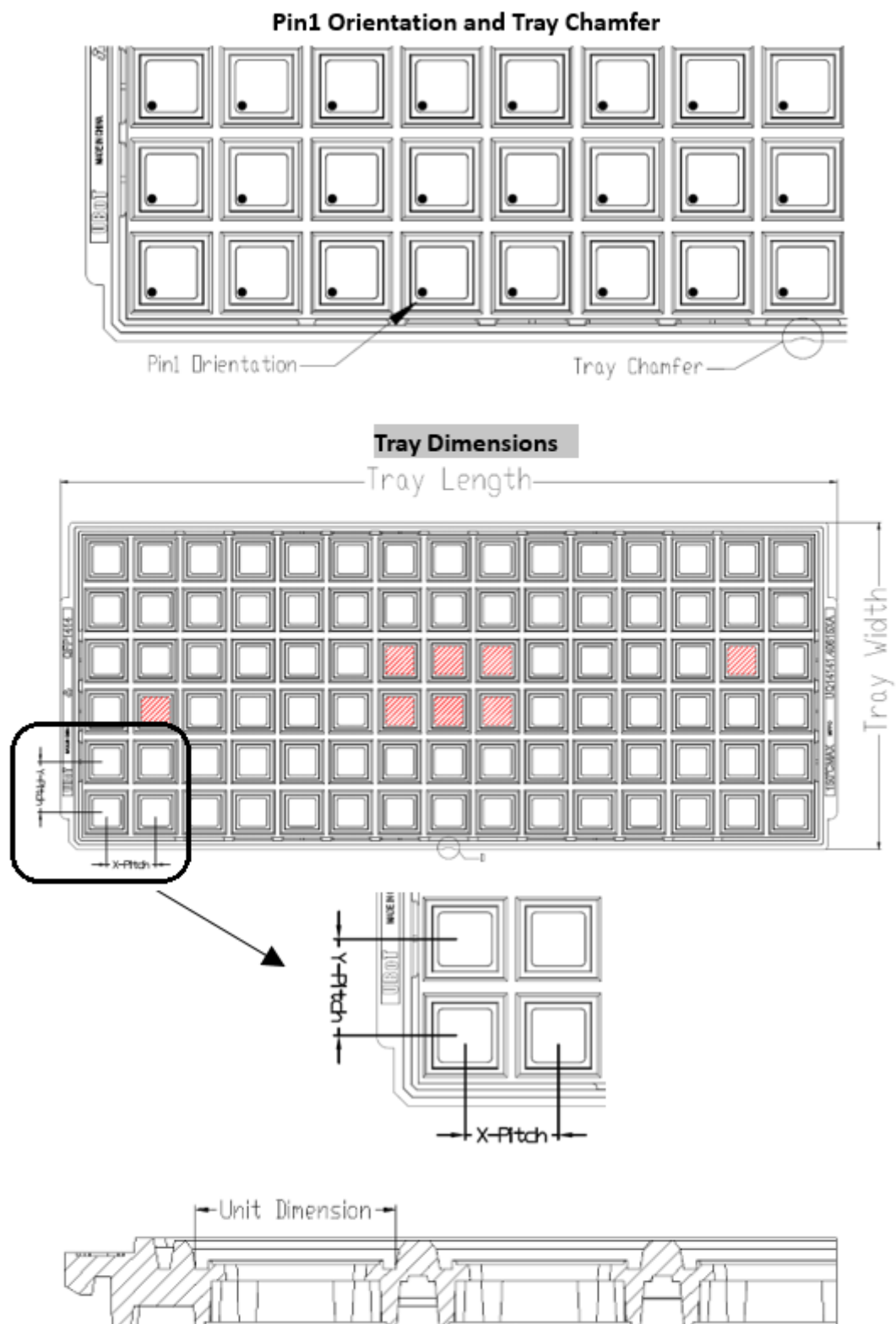
图31 托盘包装示意图
