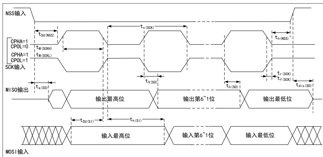
图16 SPI 时序图 — 从模式和 CPHA=1 (1)
