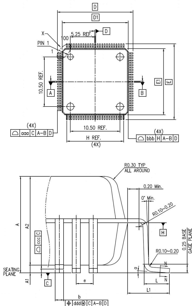
图21 LQFP100 封装图
