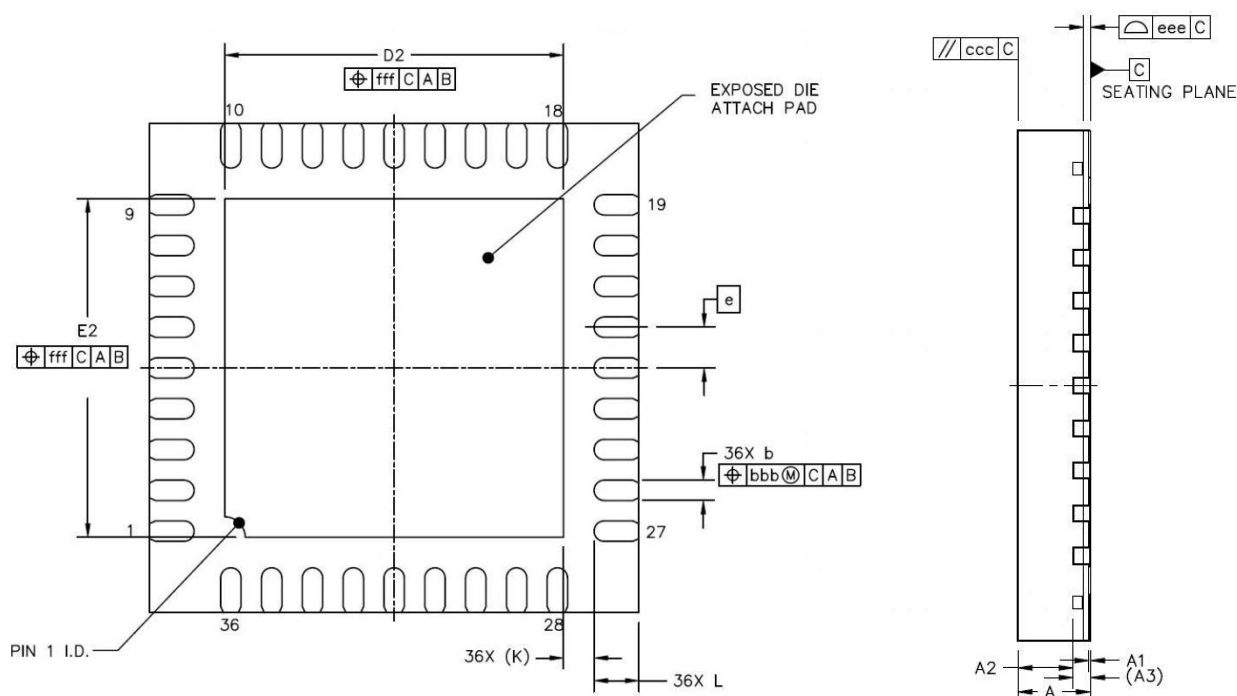
图27 QFN36 封装图
