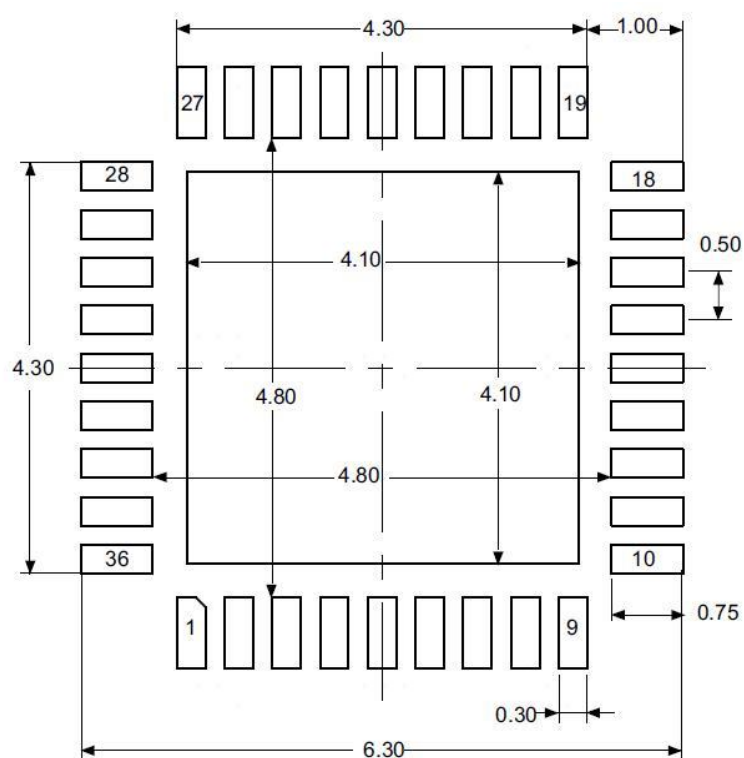
图28 QFN36 - 36 引脚，6 x 6 mm 焊接 Layout 建议
